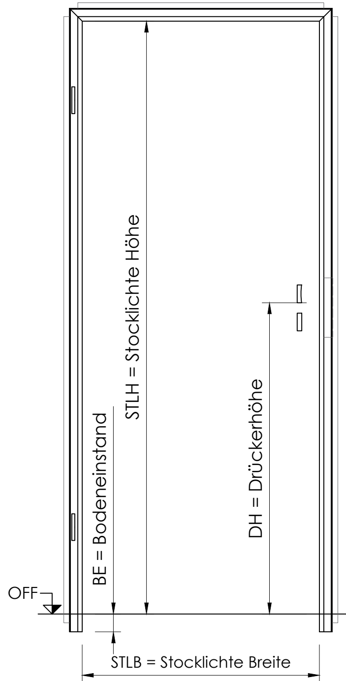
Umfassungszarge Profil 3-seitig
