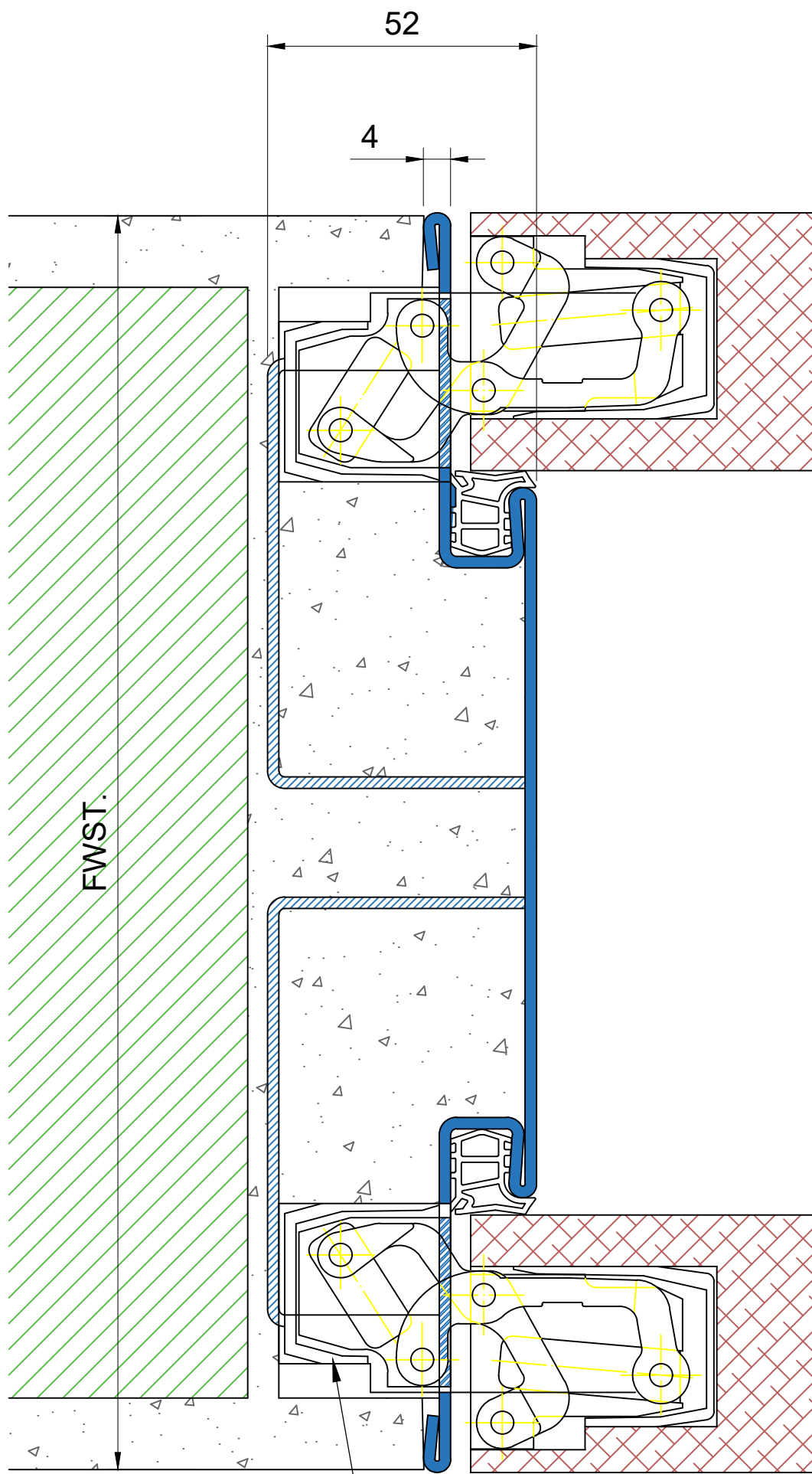
Simons TECTUS 311-3D FVZ oder Simons TECTUS 541-3D FVZ
