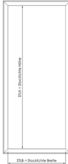
Schattennut-Durchgangszarge Profil 4-seitig
