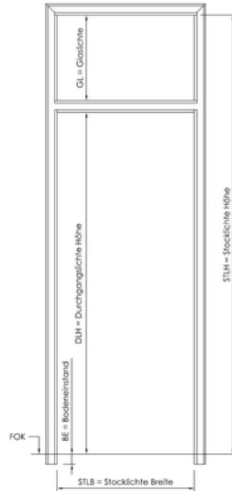
Schattennut Pendeltürzarge mit Oberlichte
