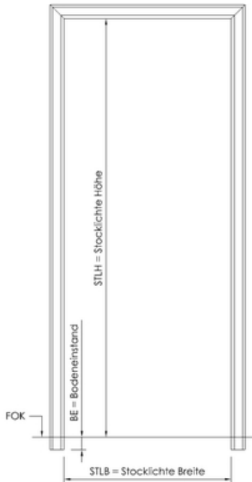
Schattennut Pendeltürzarge
