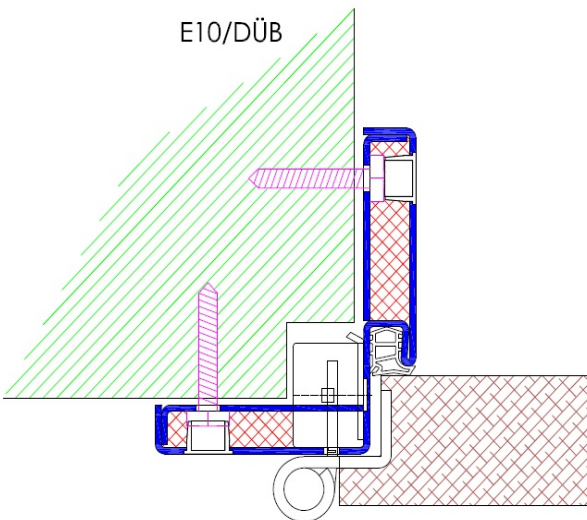
Profil E10 / Einbau mit Schraubmontage
