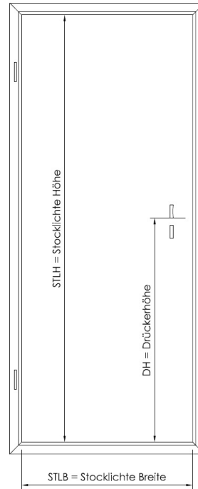
Eckzarge Profil 4-seitig
