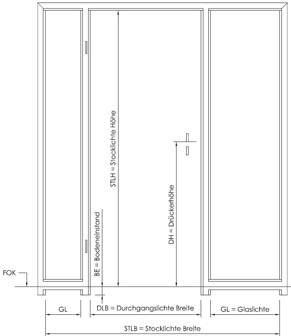
Eckzarge mit 2-facher Seitenlichte
