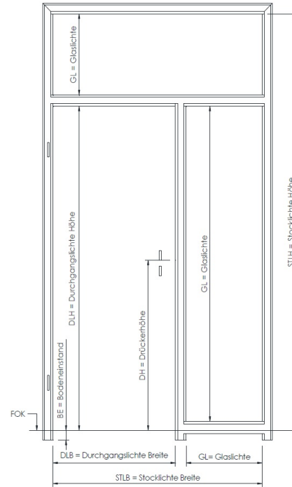
Schattentur Eckzarge mit Ober- und 2-facher Seitenlichte
