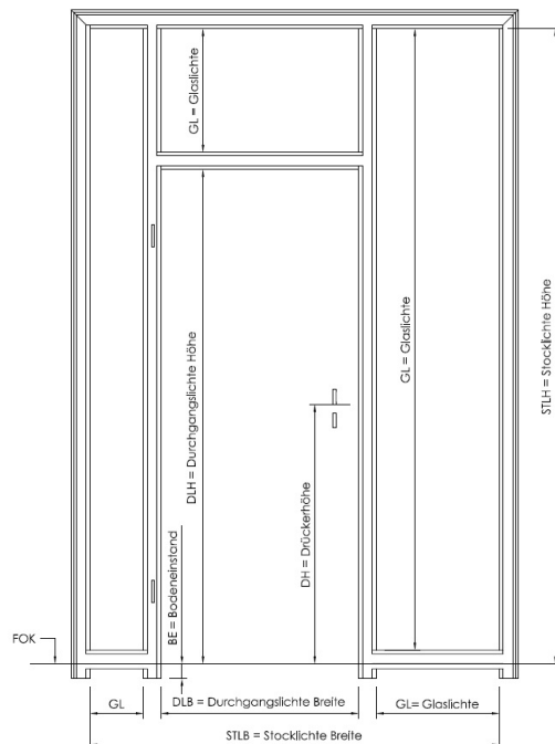
Schattennut Eckzarge mit Ober- und 2-facher Seitenlichte
