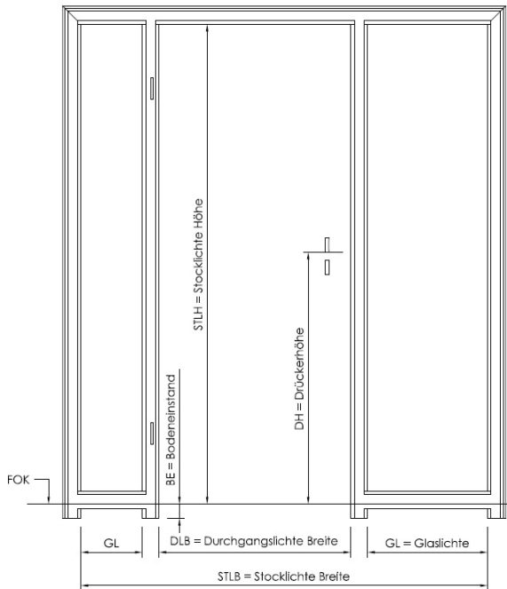
Schattennut Eckzarge mit 2-facher Seitenlichte
