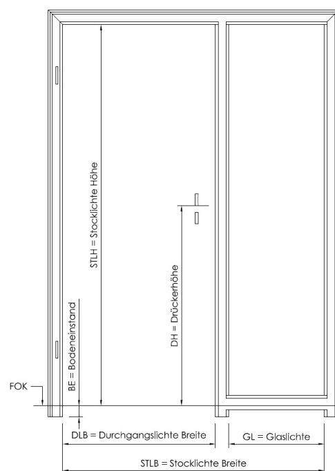
Schattennut Eckzarge mit Seitenlichte
