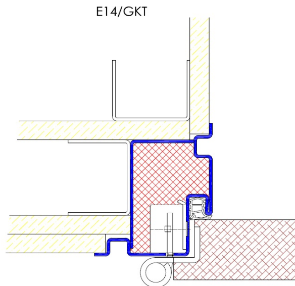
Profil E14 / Einbau in GKT-Ständerwand
