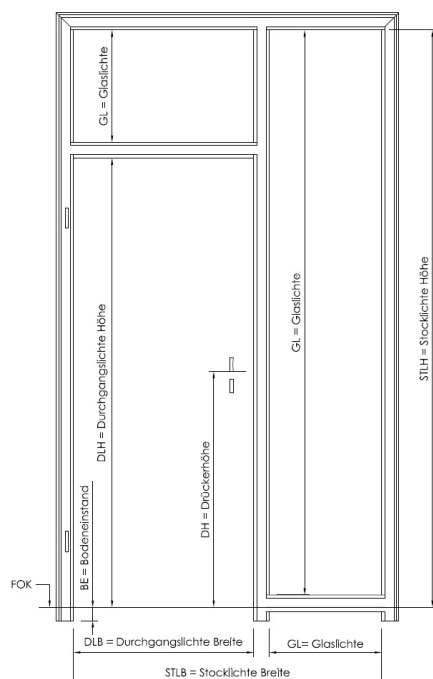
Schattennut Eckzarge mit Ober- und Seitenlichte
