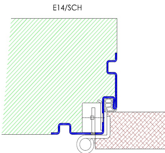
Profil E14 / Einbau in Betonschalung
