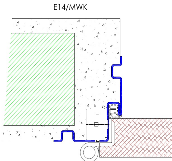
Profil E14 / Einbau in Mauerwerk
