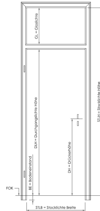
Schattennut Eckzarge mit Oberlichte
