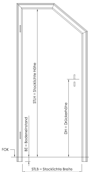
Schattennut Eckzarge mit Gehrungskopfteil
