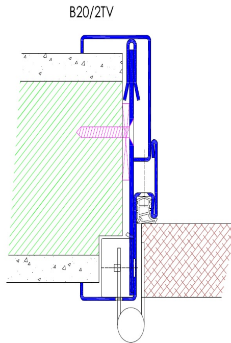
Profil B20 / 2-teilig mit verstellbarer Maulweite
