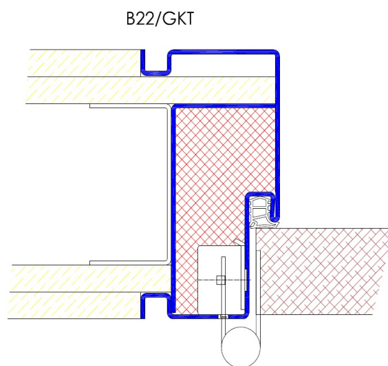
Profil B22 / Einbau in Mauerwerk
