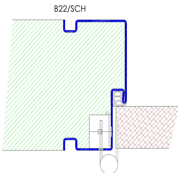
Profil B22 / Einbau in Betonschalung
