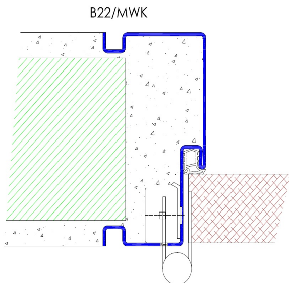
Profil B22 / Einbau in GKT-Ständerwand
