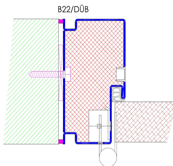
Profil B22 / Einbau mit Schraubmontage
