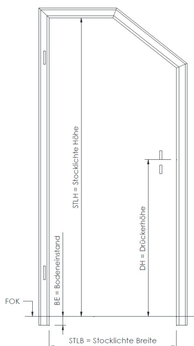
Schattennut Umfassungszarge mit Gehrungskopfteil
