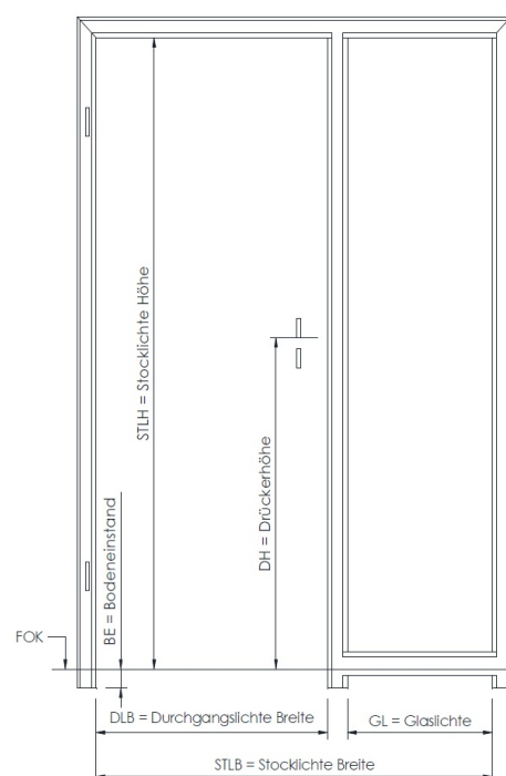
Schattennut Umfassungszarge mit Seitenlichte
