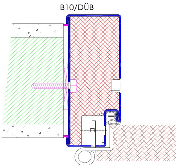
Profil B10 / Einbau mit Schraubmontage
