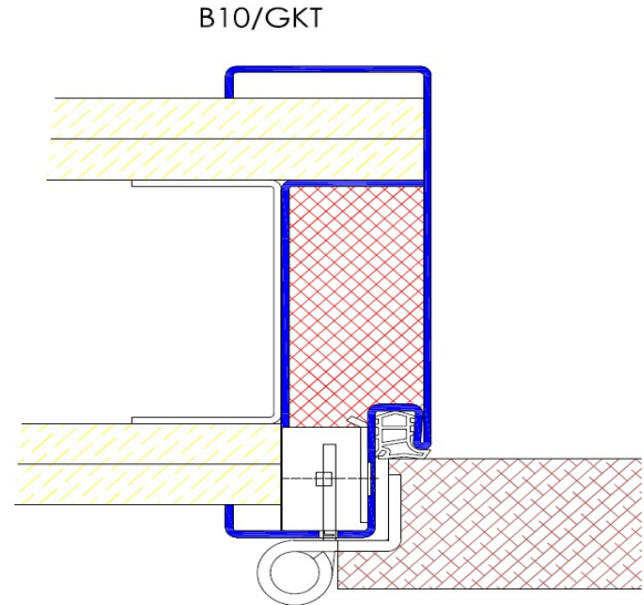
Profil B10 / Einbau in GKT-Ständerwand
