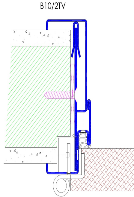
Profil B10 / 2-teilig mit verstellbarer Maulweite
