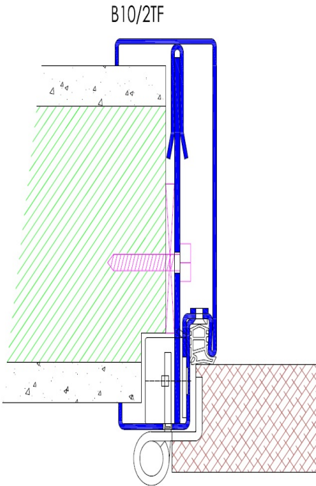
Profil B10 / 2-teilig
