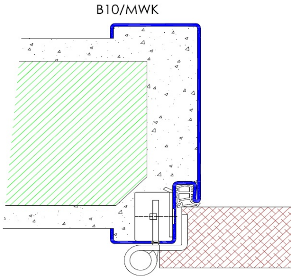
Profil B10 / Einbau in Mauerwerk
