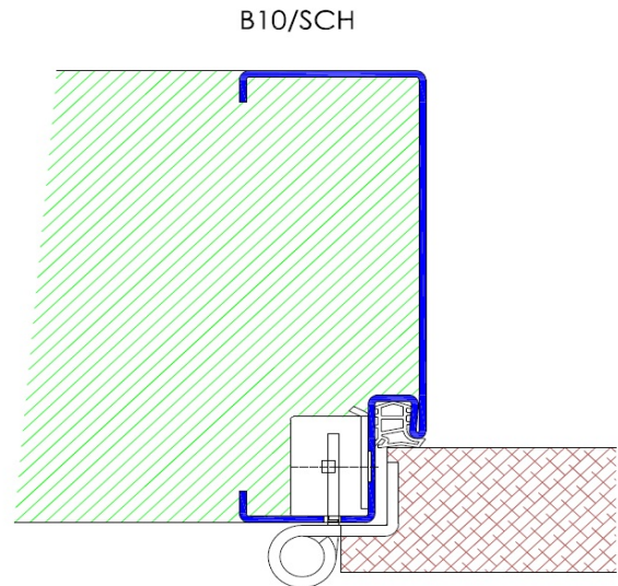
Profil B10 / Einbau in Betonschalung
