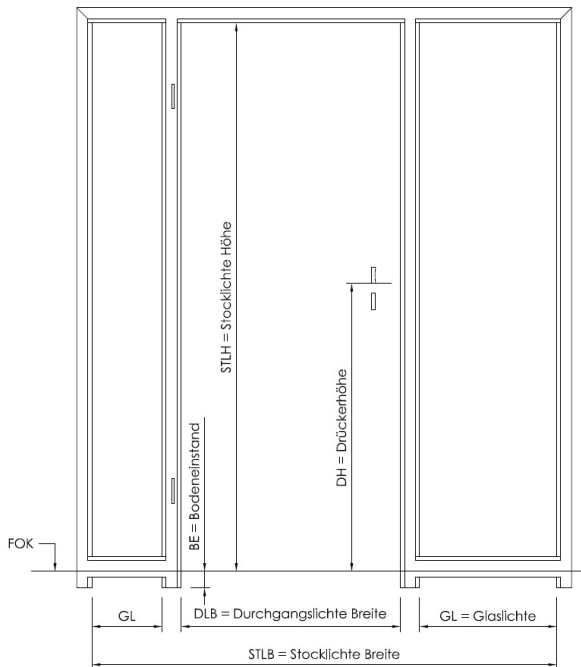
Umfassungszarge mit 2-facher Seitenlichte
