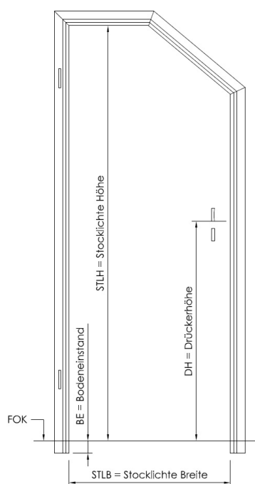
Doppelfalz-Umfassungszarge mit Gehrungskopfteil
