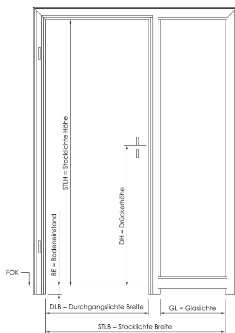
DF UZ mit Schattennut mit Seitenlichte
