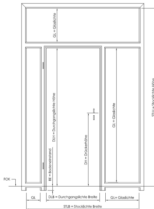
Doppelfalz-Eckzarge mit Ober- und 2-facher Seitenlichte
