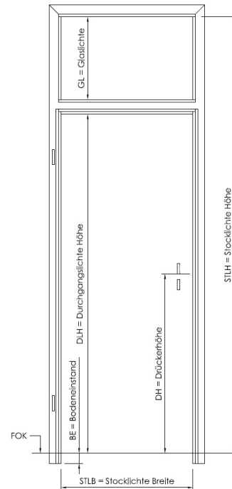
Doppelfalz-Eckzarge mit Oberlichte
