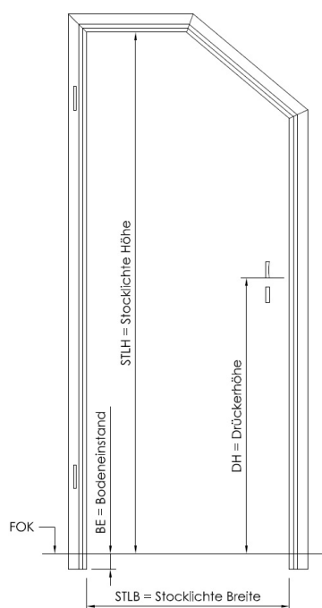
Doppelfalz-Eckzarge mit Gehrungskopfteil
