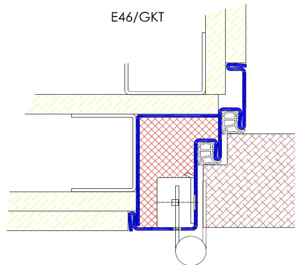
Profil E46 / Einbau in GKT-Ständerwand
