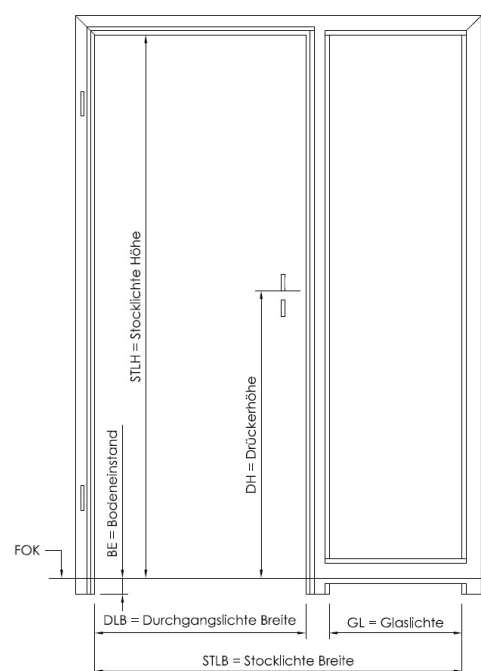
Doppelfalz-Eckzarge mit Seitenlichte
