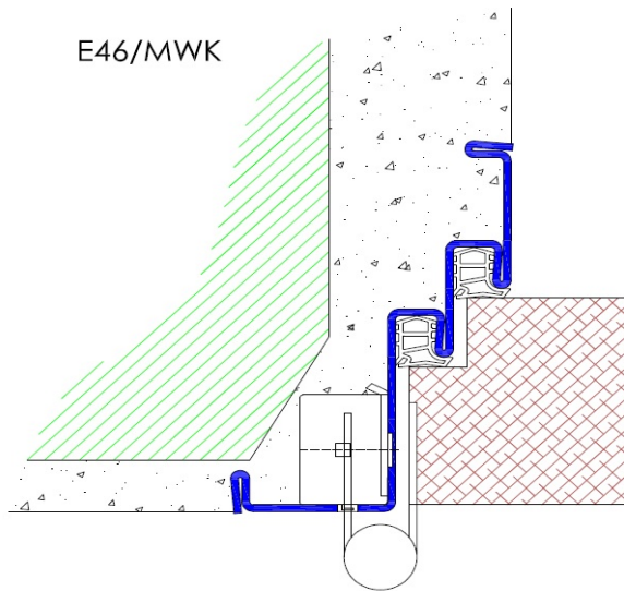
Profil E46 / Einbau in Mauerwerk
