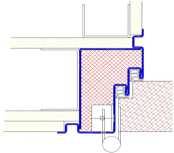
Profil E44 / Einbau in GKT-Ständerwand
