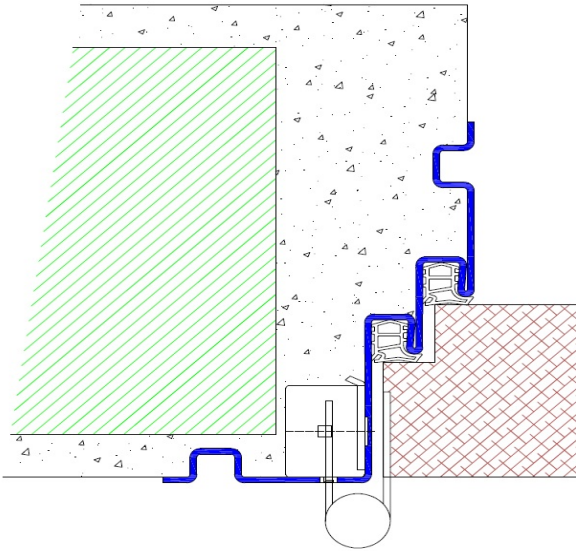
Profil E44 / Einbau in Mauerwerk
