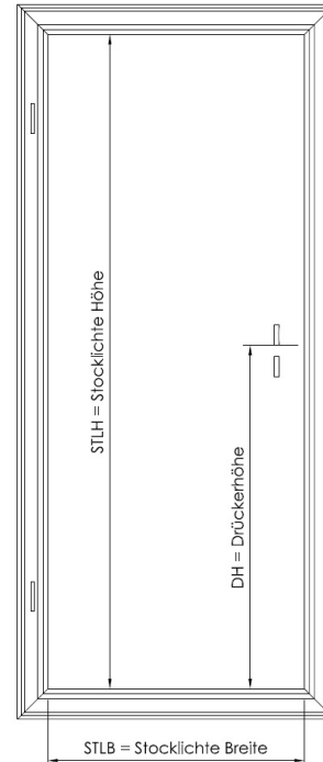
DF EZ mit Schattennut Profil 4-seitig
