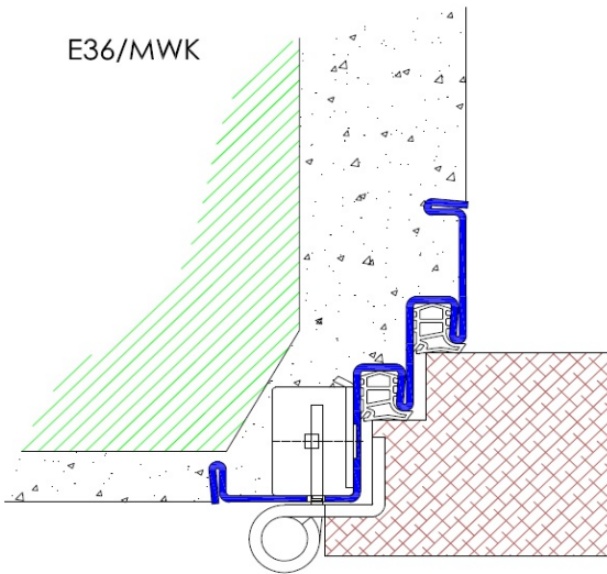
Profil E36 / Einbau in Mauerwerk
