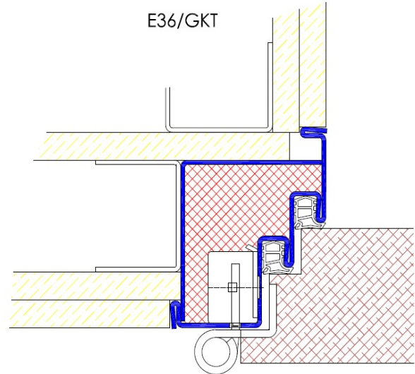
Profil E36 / Einbau in GKT-Ständerwand
