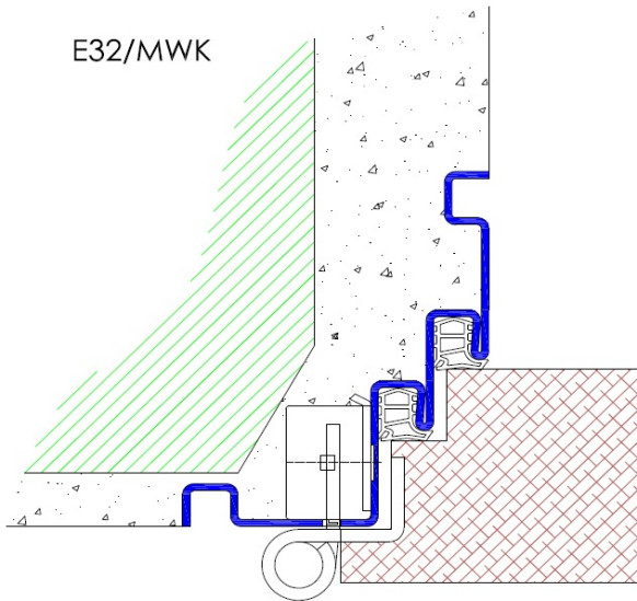
Profil E32 / Einbau in Mauerwerk
