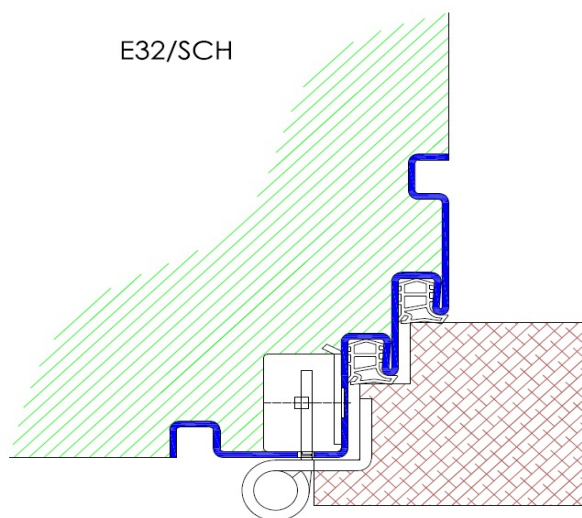
Profil E32 / Einbau in Betonschalung
