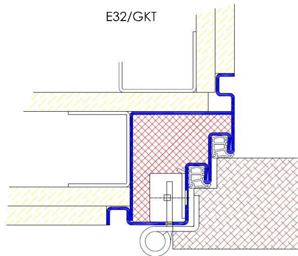
Profil E32 / Einbau in GKT-Ständerwand
