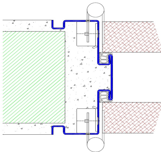
Profil Z22 / Einbau in Mauerwerk
