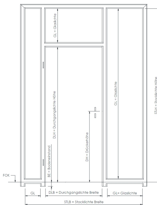
Schattennut Umfassungszarge mit Ober- und 2-facher Seitenlichte
