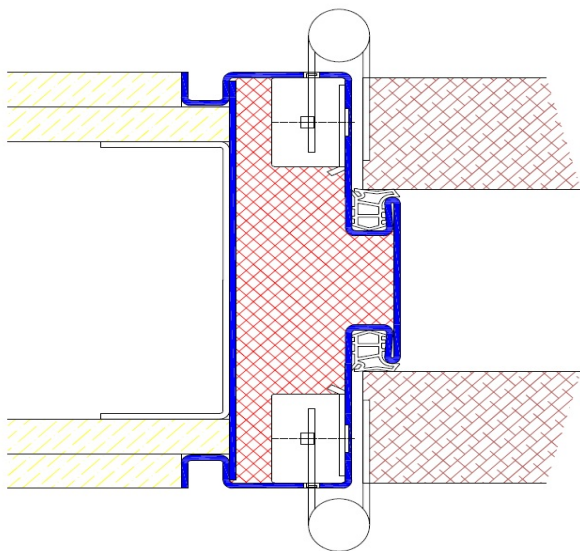
Profil Z22 / Einbau in GKT-Ständerand
