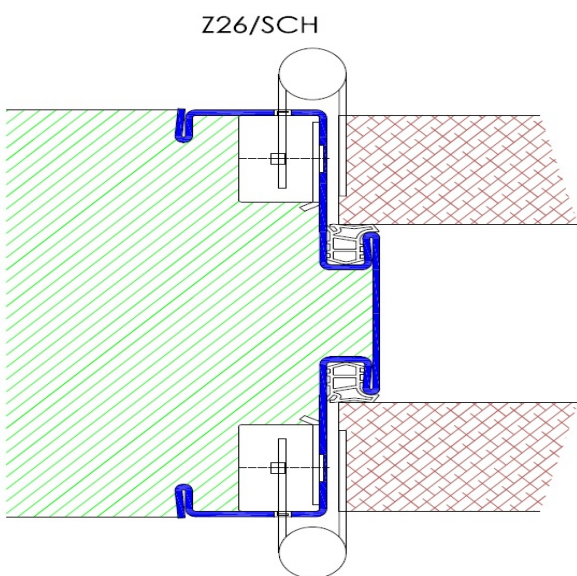
Profil Z26 / Einbau in Betonschalung Z26/SCH
