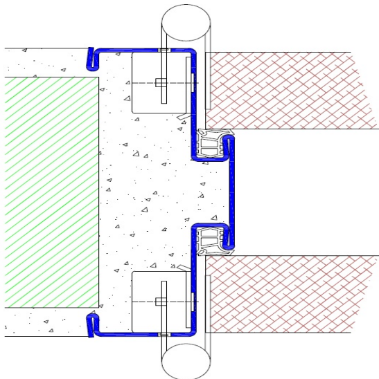
Profil Z26 / Einbau in Mauerwerk Z26/MWK
