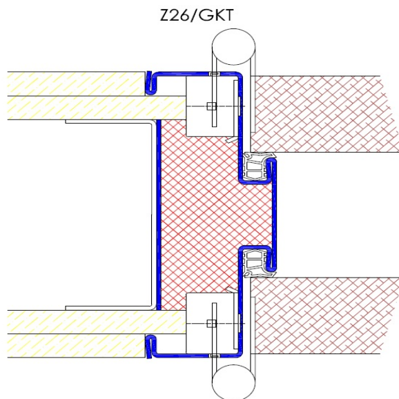
Profil Z26 / Einbau in GKT-Ständerwand Z26/GKT
