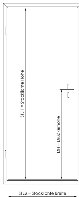
Umfassungszarge Profil 4-seitig
