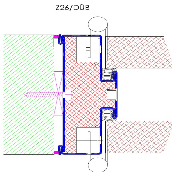
Profil Z26 / Einbau mit Schraubmontage Z26/DÜB
