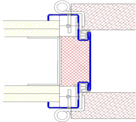
Profil Z10 / Einbau in GKT-Ständerwand
