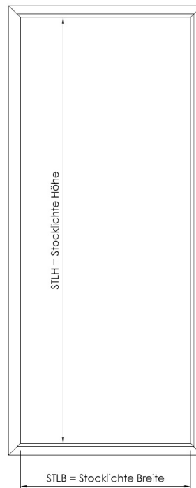
Pendeltürzarge Profil 4-seitig
