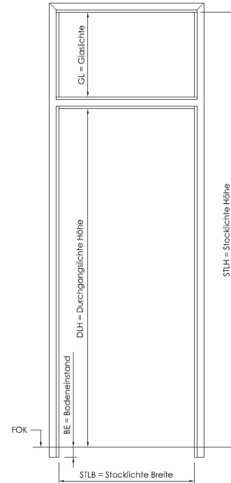
Pendeltürzarge mit Oberlichte
