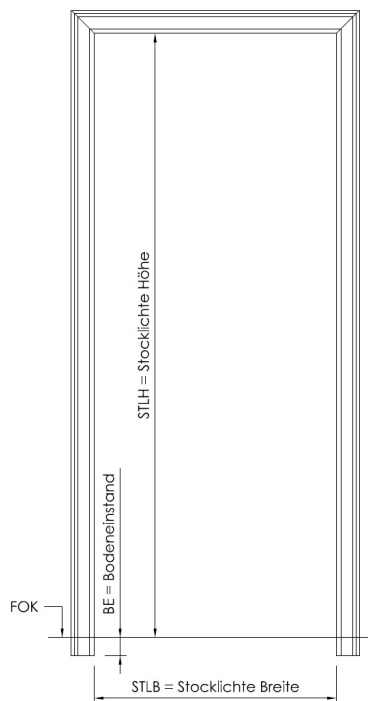
Schattennut Pendeltürzarge
