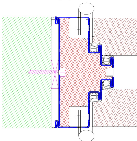
Profil Z46 / Einbau mit Schraubmontage
