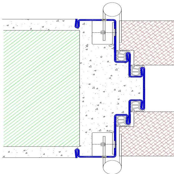
Profil Z46 / Einbau in Mauerwerk
