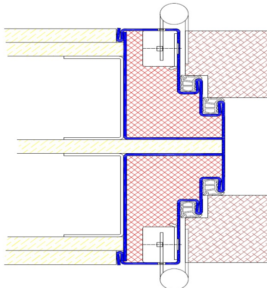
Profil Z46 / Einbau in GKT-Ständerwand
