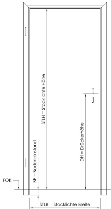
Doppelfalz-Umfassungszarge
