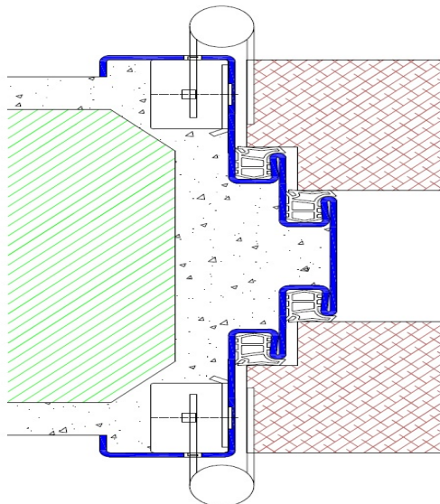
Profil Z40 / Einbau in Mauerwerk Z40/MWK
