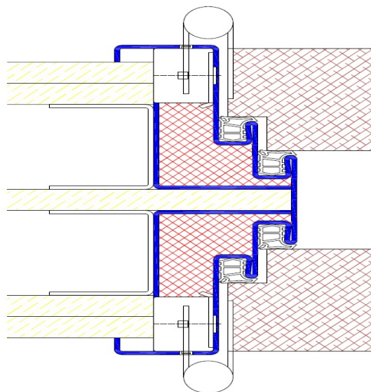
Profil Z40 / Einbau in GKT-Ständerwand Z40/GKT
