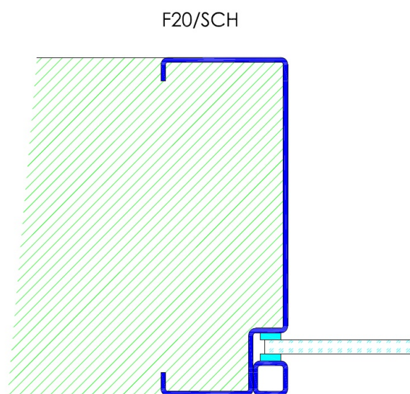
Profil F20 / Einbau in Betonschalung
