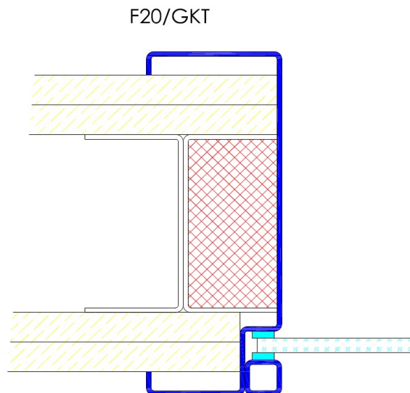
Profil F20 / Einbau in GKT-Ständerwand
