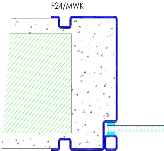
Profil F24 / Einbau in Mauerwerk
