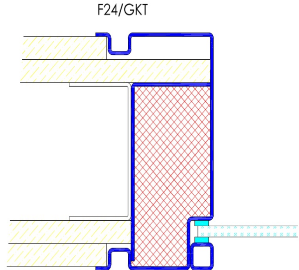
Profil F24 / Einbau in GKT-Ständerwand
