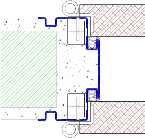
Profil Z14 / Einbau in Mauerwerk Z14/MWK
