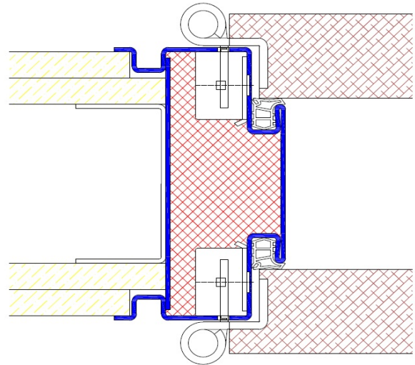
Profil Z14 / Einbau in GKT-Ständerwand Z14/GKT
