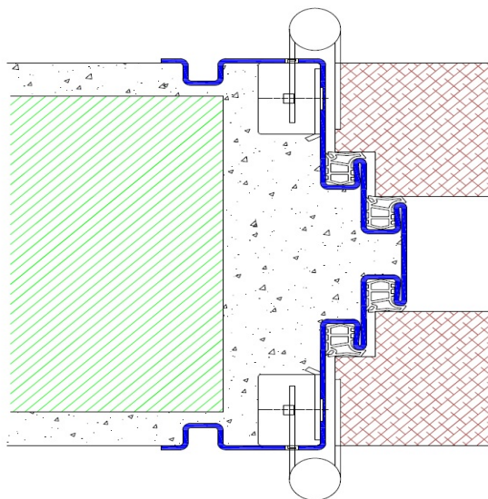
Profil Z44 / Einbau in Mauerwerk
