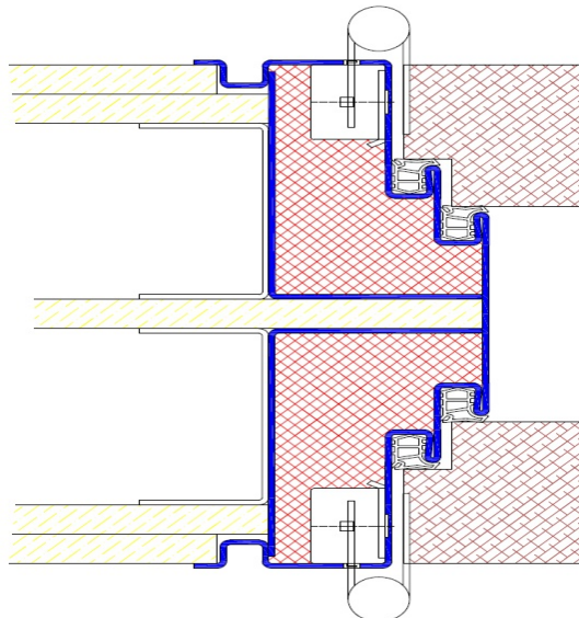
Profil Z44 / Einbau in GKT-Ständerwand
