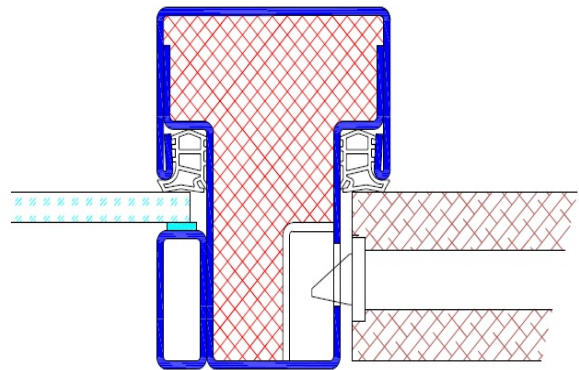
Kämpferprofil K20 mit Schlossaufnahme
