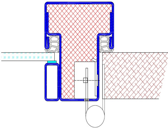
Kämpferprofil K20 mit Bandaufnahme
