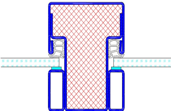
Kämpferprofil K20 beidseitig Glas
