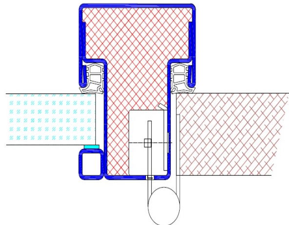
Kämpferprofil K20 mit Bandaufnahme und Isolierverglasung
