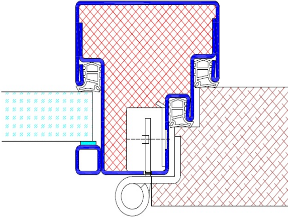
Kämpferprofil K30 mit Bandaufnahme
