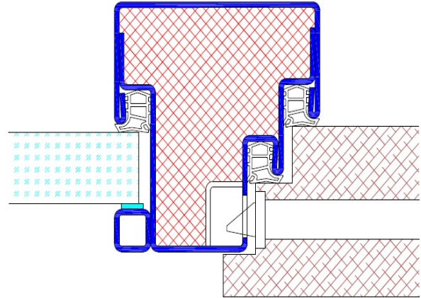
Kämpferprofil K30 mit Schlossaufnahme
