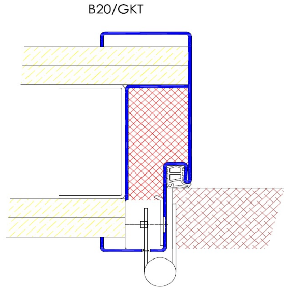
Profil B20 / Einbau in GKT-Ständerwand
