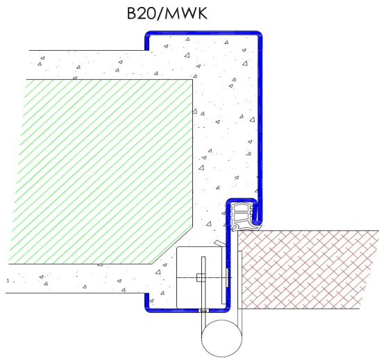
Profil B20 / Einbau in Mauerwerk
