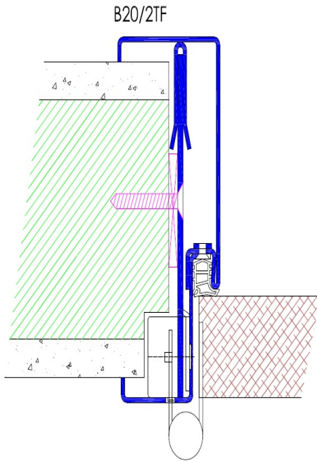
Profil B20 / 2-teilig
