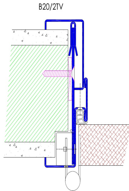
Profil B20 / 2-teilig mit verstellbarer Maulweite
