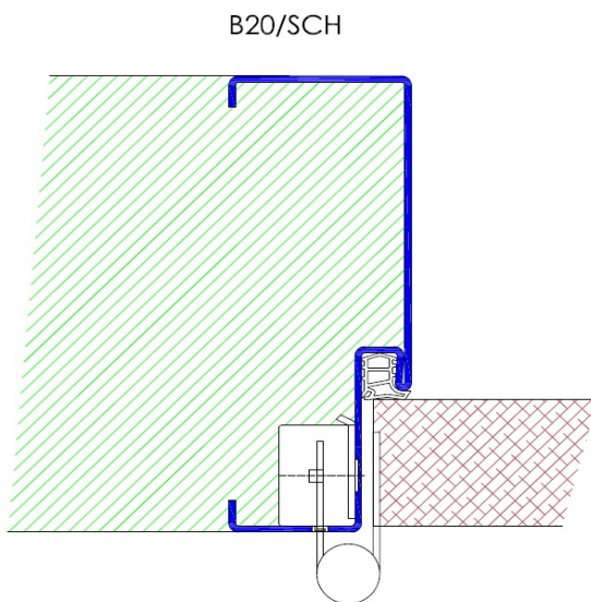
Profil B20 / Einbau in Betonschalung
